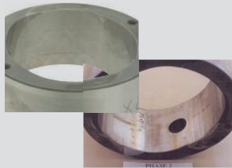
〈베인펌프 마모〉
