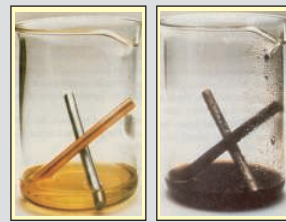
〈열안정성 차이〉
